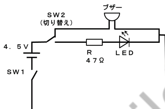
【回路図】
